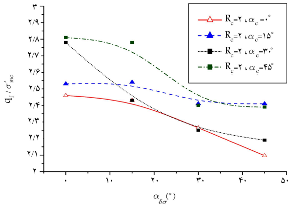
شکل ۱۶. تغییرات مقاومت برشی نسبت به \alpha_{\delta\sigma} برای نمونه‌های تحت تحکیم ناهمسان با زوایه‌های مختلف.
