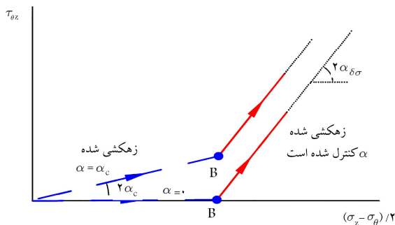
شکل ۵. مسیر تنش آزمایش‌های انجام شده بر روی نمونه‌های تحت تحکیم ناهمسان قائم و غیرقائم.
