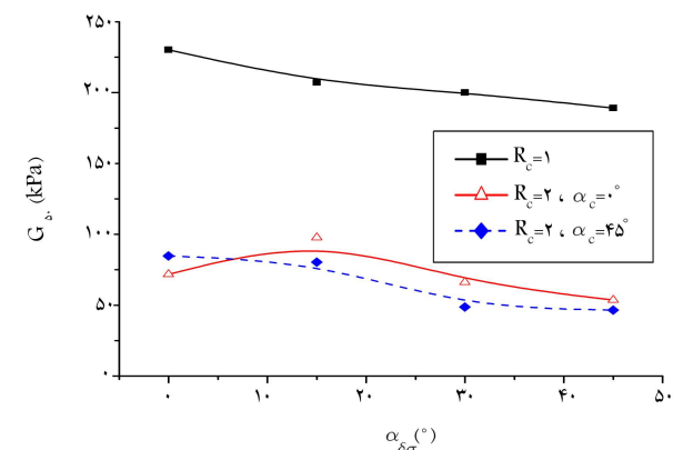
شکل ۲۳. تغییرات مدول برشی نسبت به \alpha_{\delta\sigma} برای نمونه‌های تحت تحکیم همسان و ناهمسان.
