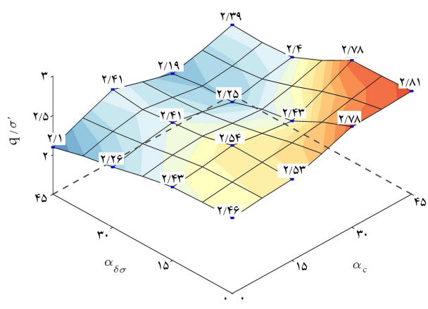
شکل ۱۸. تغییرات سه‌بعدی مقاومت برشی نسبت به \alpha_{\delta\sigma} و \alpha_c .
