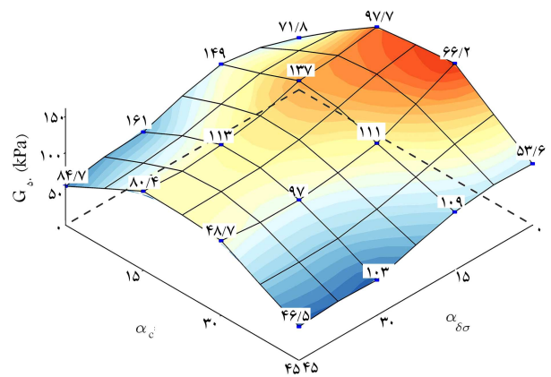
شکل ۲۲. تغییرات سه‌بعدی مدول برشی نسبت به \alpha_{\delta\sigma} و \alpha_c برای نمونه‌های تحت تحکیم ناهمسان با زاویه‌های مختلف.
