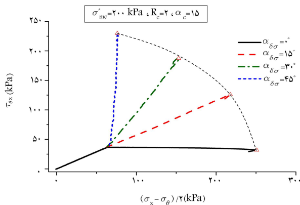
شکل ۱۱. مسیر تنش و پوش گسیختگی نمونه‌های ماسه‌بی تحت تنش‌های اولیه‌ی ناهمسان قائم با زاویه‌ی \alpha_c = 15^\circ .
