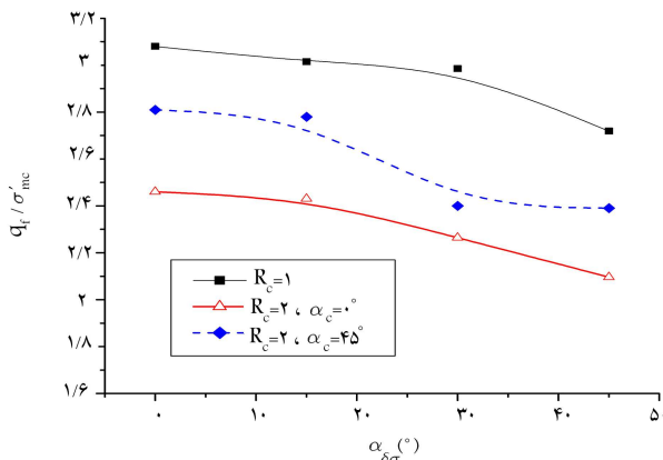
شکل ۱۷. تغییرات مقاومت برشی نسبت به \alpha_{\delta\sigma} برای نمونه‌های تحت تحکیم همسان و ناهمسان با زوایه‌های مختلف.
