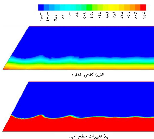
شکل ۱۳. تانک دارای یک دیواره‌ی نوسانی با زاویه‌ی 3^\circ درجه نسبت به قائم در لحظه‌ی t = 4s .
