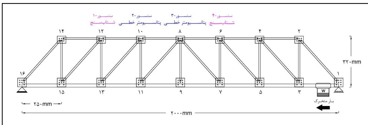
شکل ۲: شماتیک پل خرنایی
