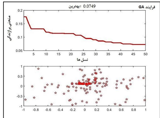
شکل ۱۳: منحنی برازندگی مربوط به عملکرد الگوریتم ژنتیک
