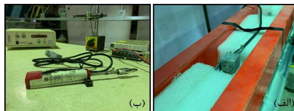
شکل ۸: الف) شتاب‌سنج (ب) پتانسیومتر خطی
