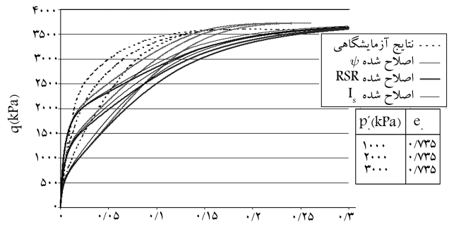
شکل ۱۰. نمودار تنش برشی در مقابل کرنش محوری، برای مقایسه‌ی داده‌های آزمایشگاه با داده‌های پیش‌بینی شده با مدل‌های اصلاح‌شده (برای ماسه‌ی Toyoura با نسبت تخلخل اولیه‌ی ۰/۷۳۵).
