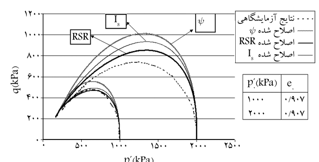
شکل ۱۱. نمودار تنش برشی درمقابل تنش میانگین مؤثر، برای مقایسه‌ی داده‌های آزمایشگاه با داده‌های پیش‌بینی شده با مدل‌های اصلاح‌شده (برای ماسه‌ی Toyoura با نسبت تخلخل اولیه‌ی ۰/۹۰۷).
