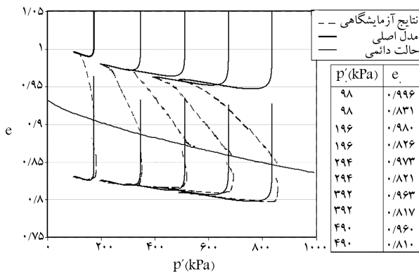
شکل ۲. نمودار نسبت تخلخل-تنش متوسط میانگین، برای مقایسه‌ی داده‌های آزمایش زهکشی شده در مقابل داده‌های پیش‌بینی شده با مدل Manzari (۱۹۹۴).
