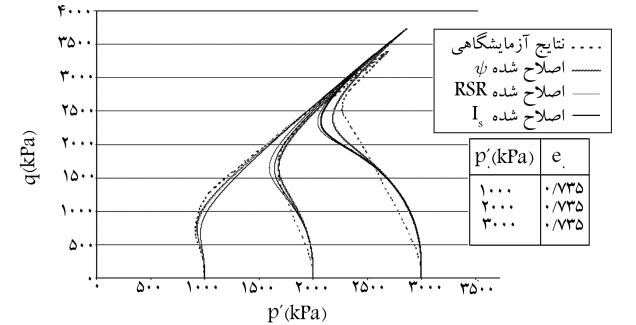
شکل ۹. نمودار تنش برشی در مقابل تنش میانگین مؤثر، برای مقایسه‌ی داده‌های آزمایشگاه با داده‌های پیش‌بینی شده با مدل‌های اصلاح‌شده (برای ماسه‌ی Toyoura با نسبت تخلخل اولیه‌ی ۰/۷۳۵).
