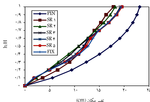
شکل ۱۷. تغییر مکان طبقات تحت رکورد زلزله‌ی چی - چی با مدل‌های سازه‌ی مختلف.
