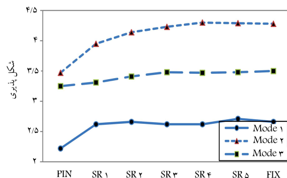
شکل ۱۰. تغییرات شکل‌پذیری نسبت به صلبیت اتصال.
