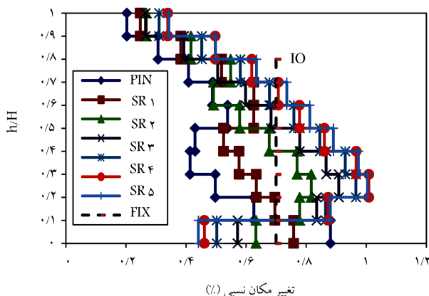
شکل ۲۷. مقایسه‌ی جابه‌جایی نسبی مدل‌های سازه‌یی تحت رکورد کبه.
