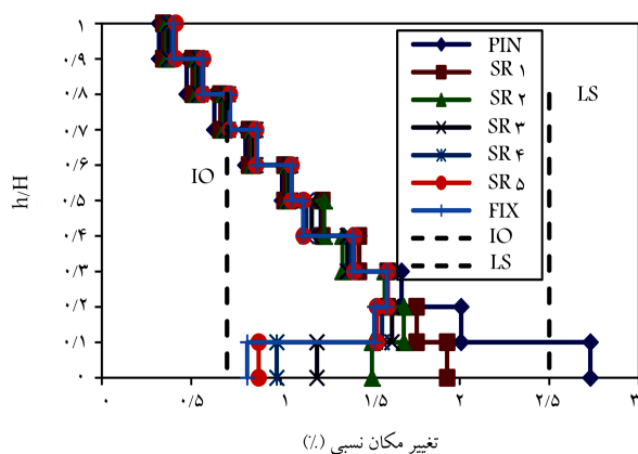
شکل ۲۳. مقایسه‌ی جابه‌جایی نسبی مدل‌های سازه‌یی تحت رکورد مصنوعی تولید شده مطابق رکورد چی - چی با روش MPA.
