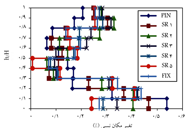
شکل ۳۲. مقایسه‌ی جابه‌جایی نسبی مدل‌های سازه‌ی تحت رکورد نورث‌ریج.
