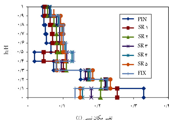
شکل ۳۴. مقایسه‌ی جابه‌جایی نسبی مدل‌های سازه‌ی تحت رکورد سان‌فرانسیسکو.
