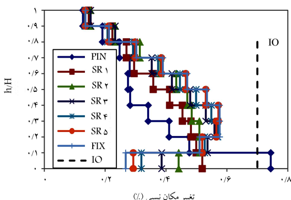
شکل ۲۵. مقایسه‌ی جابه‌جایی نسبی مدل‌های سازه‌یی تحت رکورد کوالینگا.
