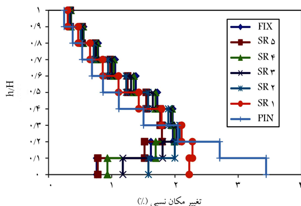
شکل ۲۲. مقایسه‌ی جابه‌جایی نسبی مدل‌های سازه‌یی تحت رکورد مصنوعی تولید شده مطابق شرایط ساختگاهی با روش MPA.
