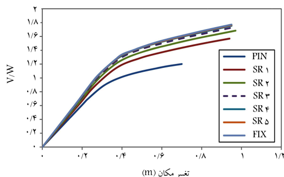
شکل ۷. مقایسه‌ی منحنی‌های ظرفیت برای مدل‌های مختلف برای مود اول.
