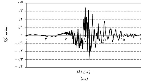
شکل ۲. رکورد زلزله‌های مصنوعی تولید شده.
