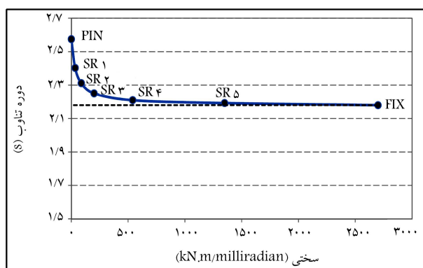
شکل ۴. تغییرات دوره تناوب مود اول براساس سختی پای ستون.
