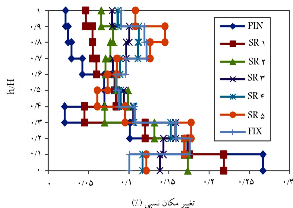
شکل ۳۳. مقایسه‌ی جابه‌جایی نسبی مدل‌های سازه‌ی تحت رکورد ویترو.
