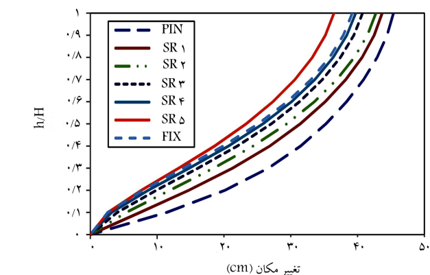
شکل ۲۴. مقایسه‌ی تغییر مکان مدل‌های سازه‌یی تحت رکورد مصنوعی تولید شده مطابق رکورد چی - چی با روش MPA.
