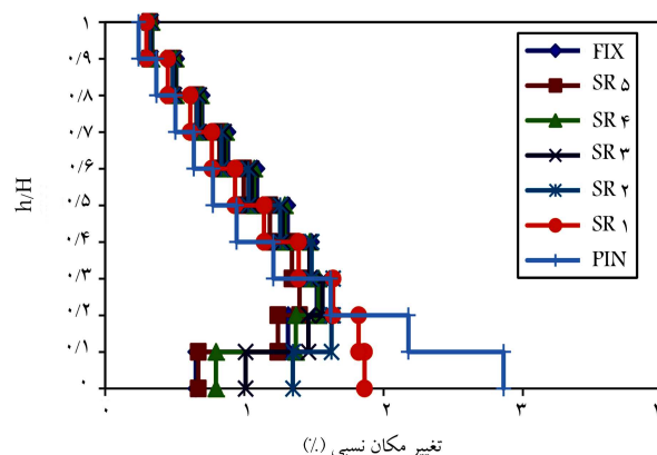
شکل ۲۶. مقایسه‌ی جابه‌جایی نسبی مدل‌های سازه‌یی تحت رکورد مصنوعی تولید شده مطابق رکورد چی - چی با روش MPA.
