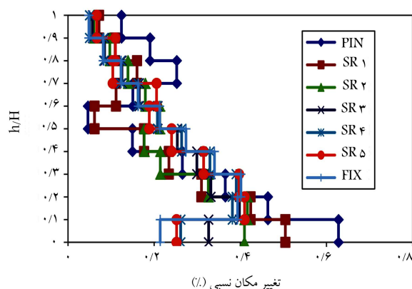
شکل ۳۱. مقایسه‌ی جابه‌جایی نسبی مدل‌های سازه‌ی تحت رکورد طُبِس.
