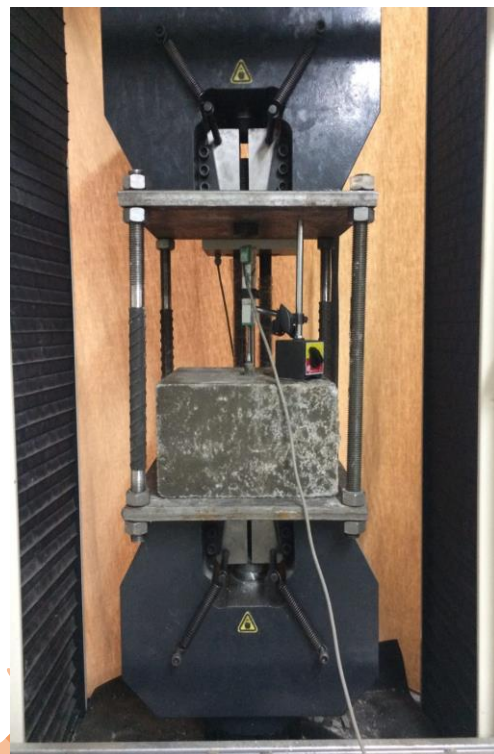
شکل ۴: آزمایش بیرون کشیدگی میلگرد و نحوه قرارگیری سنسور جابه‌جایی سنج
