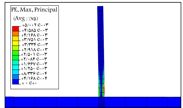
شکل ۶. کانتورکنش خمیری ایجادشده در سازه تحت اثر رکورد نورت ریج - ۰۱.
