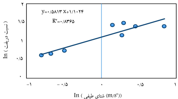
شکل ۷. تغییرات لگاریتم بیشینه‌ی نسبت دررفت ایجادشده در سازه در مقابل لگاریتم شتاب طیفی.
