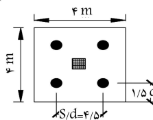
ب) مشخصات کلاهک شمع.
